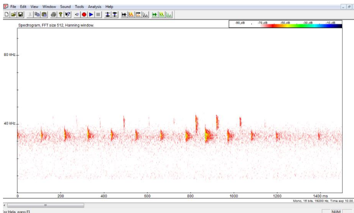
Figure 1 : Exemple de spectrogramme représentant les signaux sonars émis par une Barbastelle d'Europe sur le logiciel Batsound
